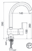
6303 Yüksek Lavabo Bataryası Basin Mixer
